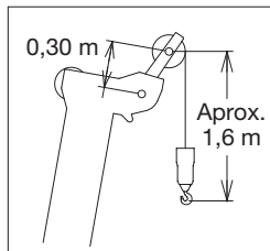
ROLDANA AUXILIAR
